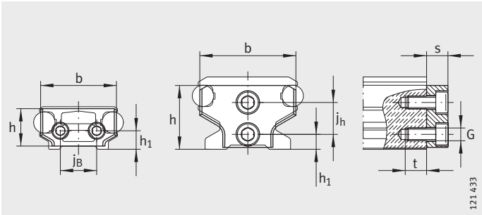
ANS.LFS
