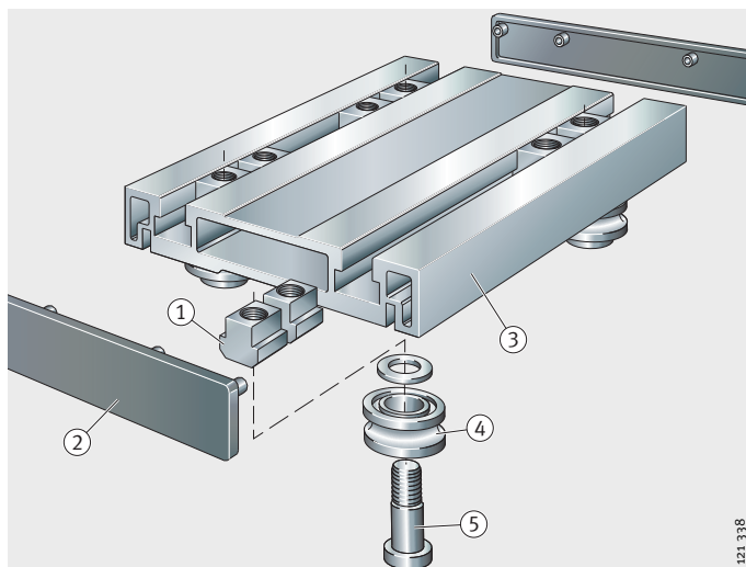
Рис. 1 Полые каретки
