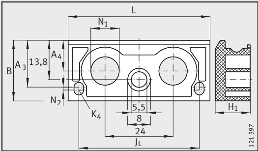
AB.LFL20
