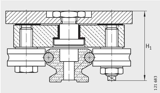
LFDL-B
