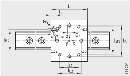
LFLL с LFS, -C, -CE, -CEE, -E, -EE, -N, -NZZ, -M, -F, -FE Вид повернут на 90°
