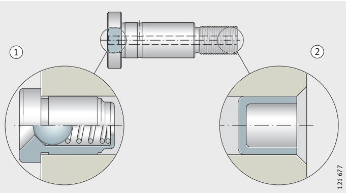
Рис. 1 Пресс-маслёнка заглушка
