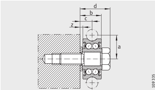
Схема установки
