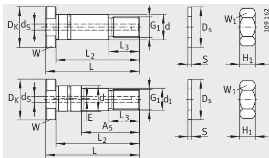
LFZ...A1, LFE...A1
