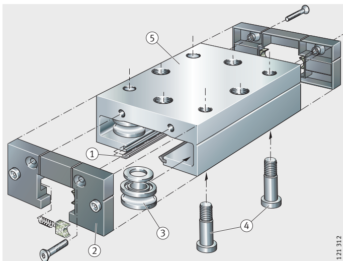
Рис. 2 Компактная каретка
