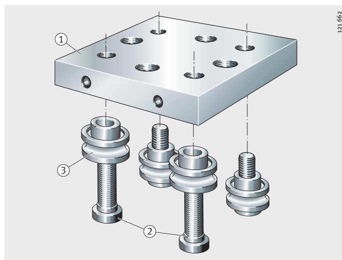
Рис. 3 Открытая каретка
