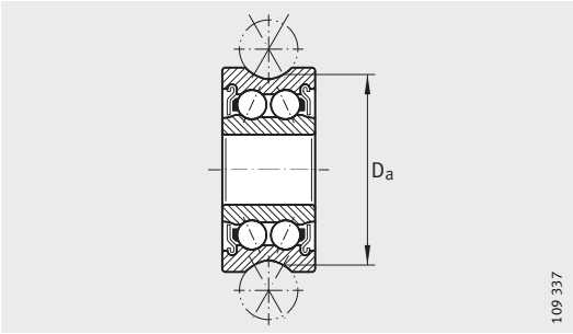
LFR...2Z
