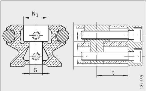
ANS.LFS..-C (полые)
